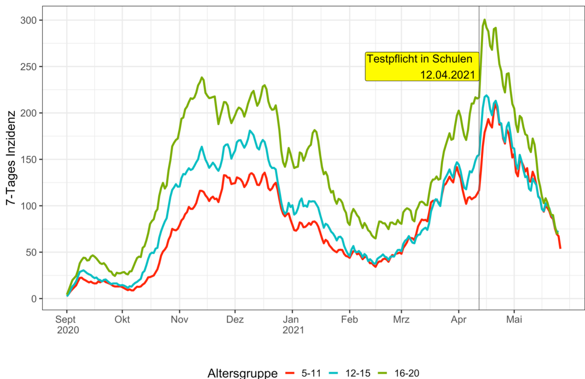
Abbildung 1.1 Altersspezifische Inzidenzen
