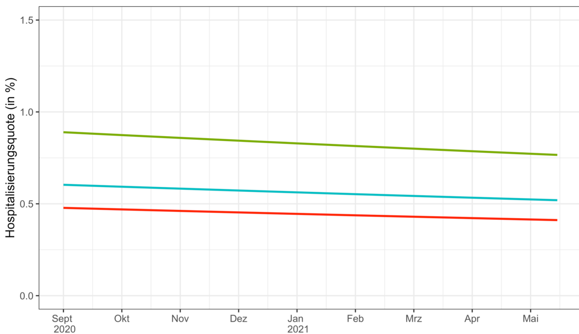
Abbildung 1.3. Hospitalisierungsquote
